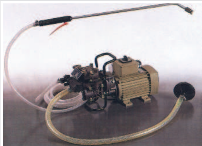
Škropilnica BM20/15-1F, stabilna Prskalica BM20/15-1F, stabilna
